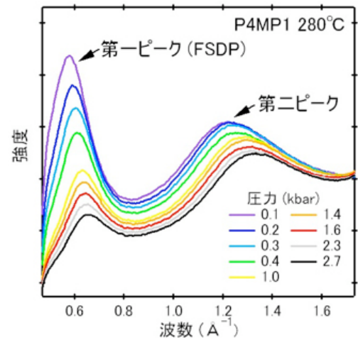
図2. P4MP1の溶融体のX線回折パターンの圧力変化
