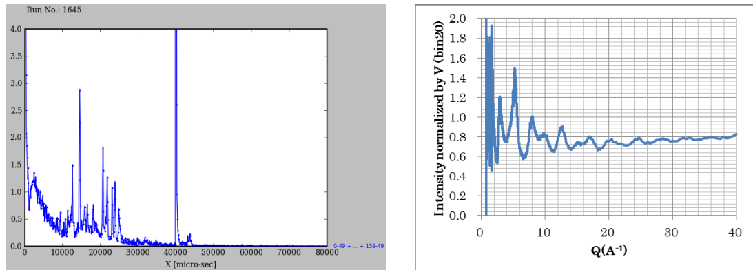
図3 (左) V-Niキャピラリー(6φ)に入れたmicaの回折パターン。(右)Vで規格化した石英ガラスのパターン。左図中央部の巨大なピークおよび右図 Q \sim 1.5 \text{ \AA}^{-1} 付近の落ち込みは、間引いた2発目のFrameのバースト中性子による影響(T0チョッパーは故障中で使えないので、その影響は甚大! )。
