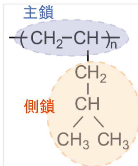
図1. P4MP1の構造式
