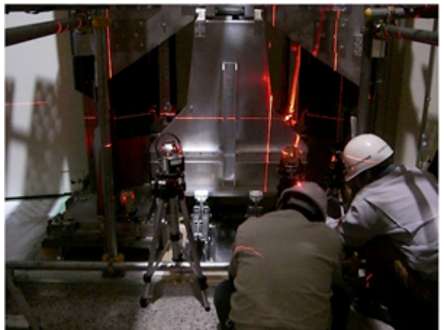
図2 据付調整中の検出器架台
