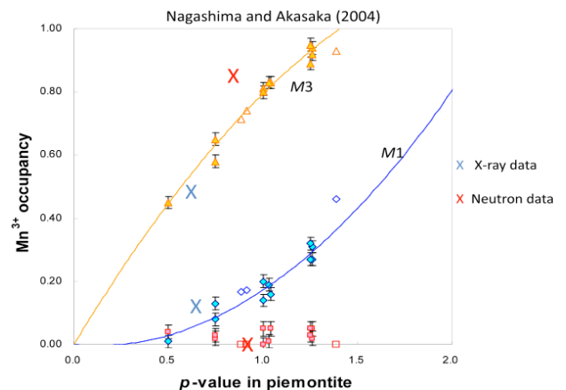
第2図 6配位席M1, M3席におけるMn 3+ の占有率。青および赤のxはそれぞれX線および中性子回折データによる結果。
