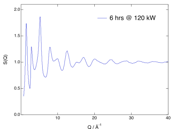
図2. 6時間の測定を行った \text{SiO}_2 ガラスの S(Q) 。J-PARC陽子加速器の運転パワーは120kW。
