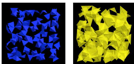
図1 RMC法により得られた Mg_2SiO_4 ガラスの構造モデル
