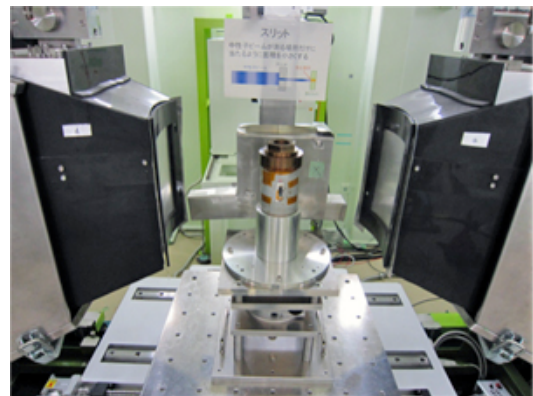
パールキュービックアンビルセルを用いた測定の様子。セルの中には補正データ測定用のバナジウムが仕込んである。
