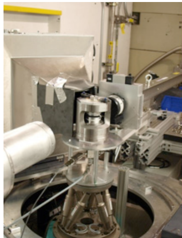
図2 SNAPにおける実験の様子。中央にパリーエジンバラセル、左手に検出器。右奥のミラーにより集光した中性子ビームがセル内の試料へと照射される。
